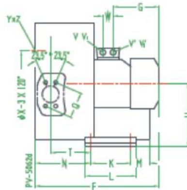
*Medidas del Soplador Regenerativo Boss Tech.
