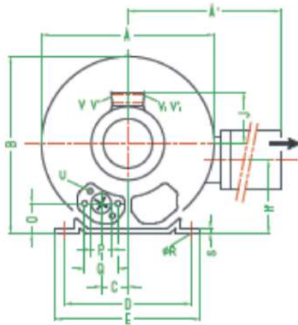
*Medidas del Soplador Regenerativo Boss Tech.
